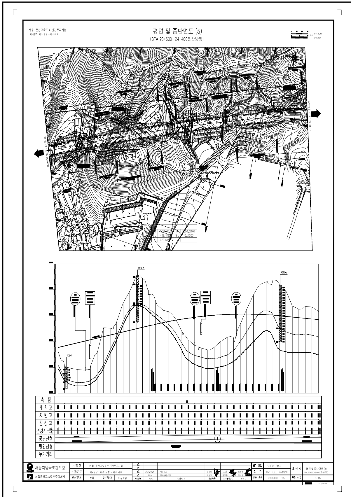
【그림 7.1.4】 종평면도
